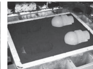
砂型 / 中子型
